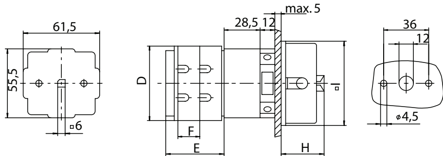
Abmessungen / Dimensions Bauform / Design: 1504/1505
